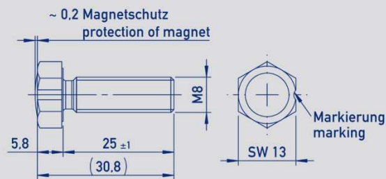
Z-RFC-P19 スクリューポジションマーカ
