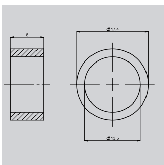
リングポジションマーカ- Z-TH1-P30, P/N 400106139
