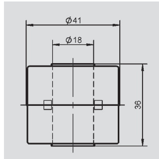
シリンダー浮動式ポジションマーカー Z-TH1-P21, P/N 400056044
