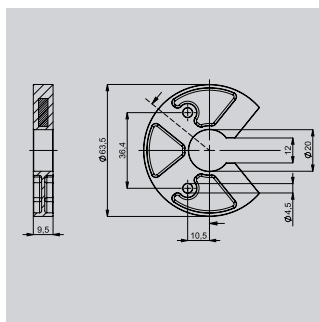
U字型ポジションマーカ- Z-TH1-P25, P/N 400105076
