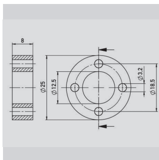
リングポジションマーカ- Z-TH1-P18, P/N 400005697
