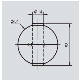
ボールタイプポジションマーカー Z-TH1-P22, P/N 400056045
