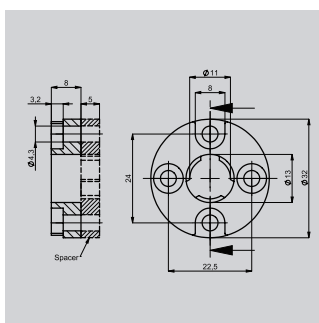
リングポジションマーカ- Z-TH1-P19, P/N 400005698
